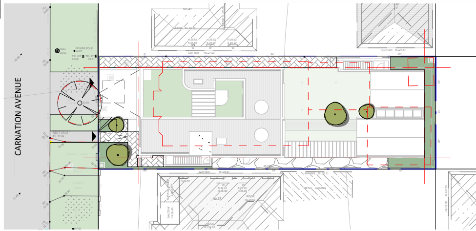
1 SITE / DEMOLITION PLAN 1 : 500
